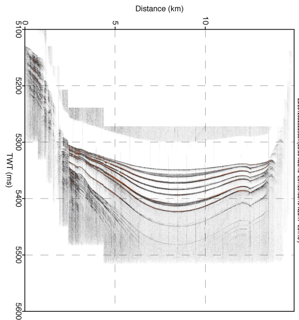
Profil OWEN 25-3b : Profil au travers du bassin N20° montrant son remplissage turbiditique et sa faille bordière principale.
